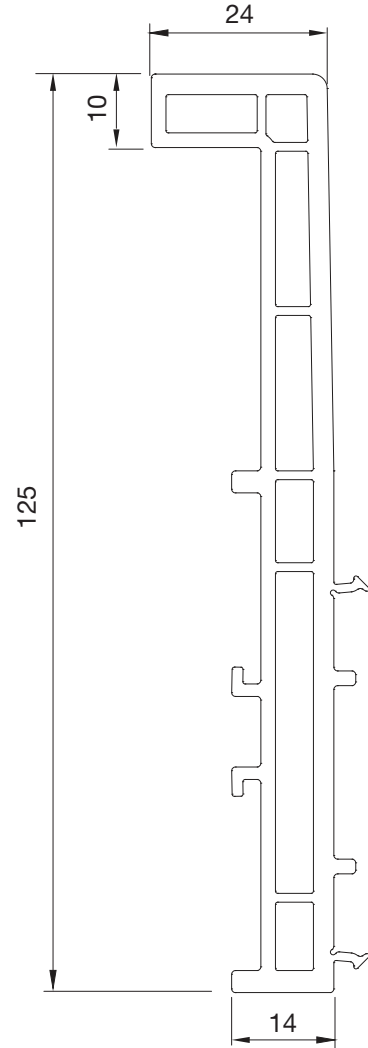
PRVN43 PERVAZ PROFİLİ CASING PROFILE
