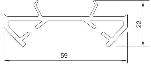
PEX2760BY.0003 KÖŞE DÖNÜŞ ADAPTÖRÜ CORNER ADAPTER
