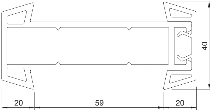
PEX2860BY.0003 KÖŞE DÖNÜŞ ADAPTÖRÜ CORNER ADAPTER
