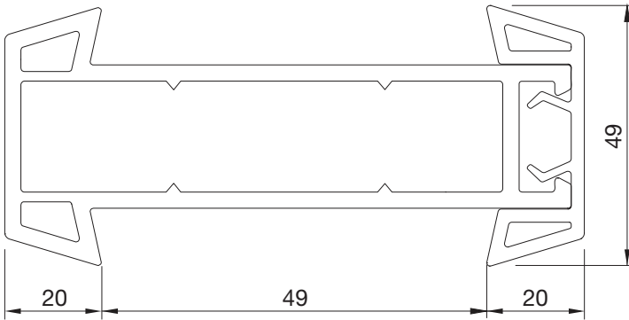
PEX2860BY.0003 KÖŞE DÖNÜŞ ADAPTÖRÜ CORNER ADAPTER
