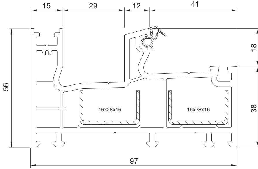
PSY4665BY.0002 FIX KASA FIX FRAME
